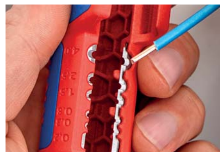
Abisolieren von Einzelleitern
