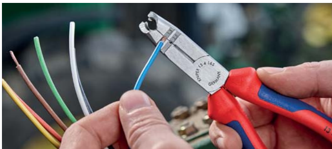
Abisolierlöcher für Leiter 1,5 und 2,5 mm 2
