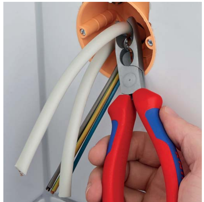
Abmanteln tief unten in der Unterputzdose
