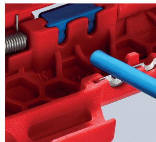
Praktische Positionierhilfe erleichtert das Einlegen von Einzelleitern zum Abisolieren
