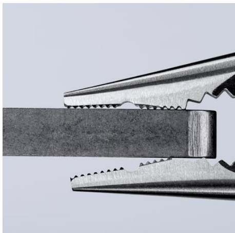
sicherer Griff auch an Flachteilen durch Dreipunktauflege
